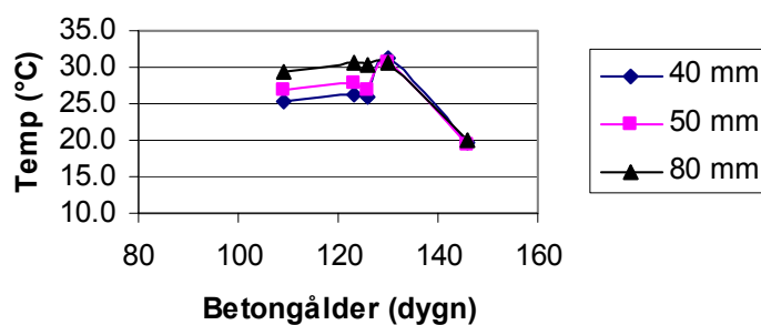
Betongtemperatur Rum 1:3
