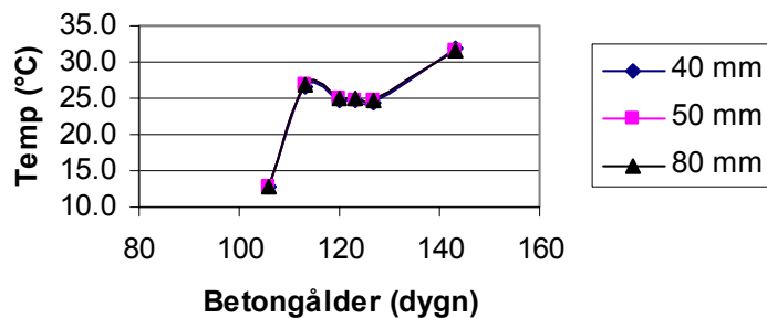
Betongtemperatur Rum 1:8
