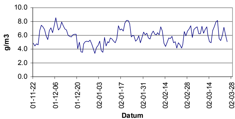
Ånghalt Rum 1:19
