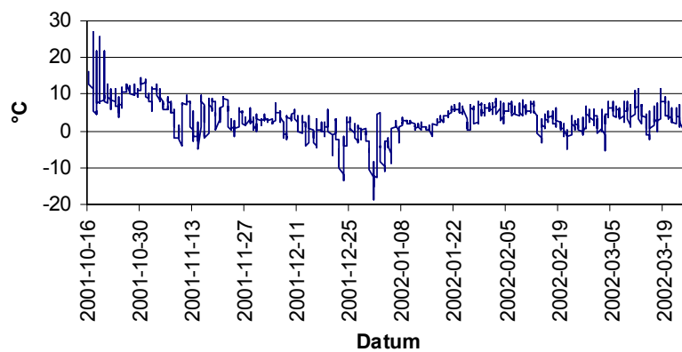
Utomhusluftens temperatur
