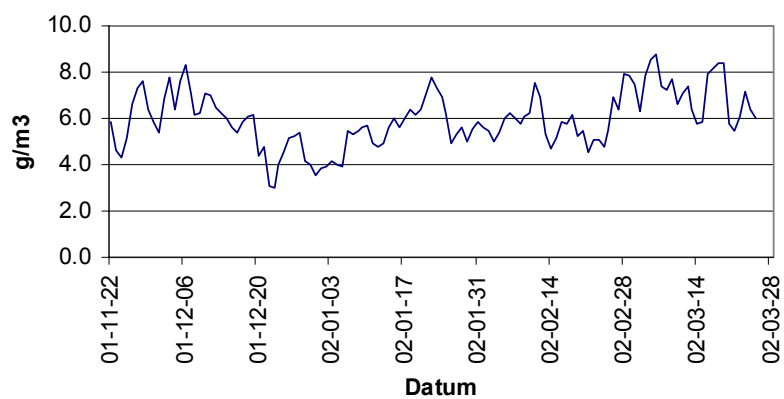
Ånghalt Rum 1:5
