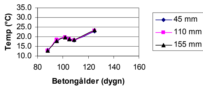
Betongtemperatur Rum 2:7
