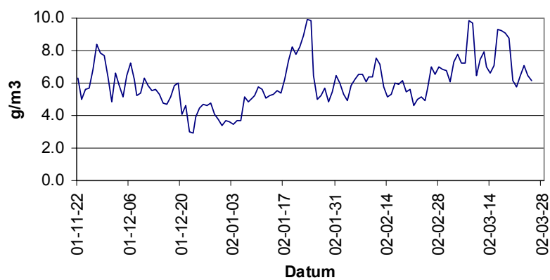
Ånghalt Rum 1:7
