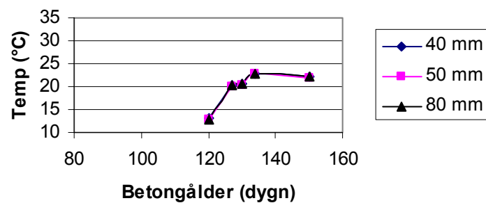
Betongtemperatur Rum 1:28
