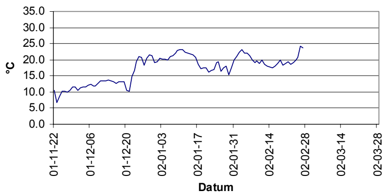
Temperatur Rum 1:13
