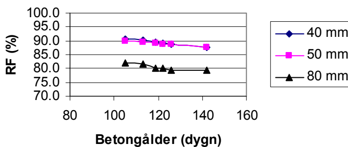
Betong-RF Rum 1:4
