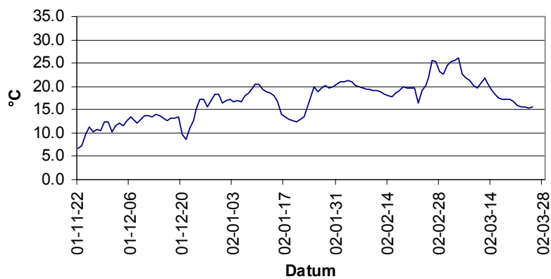
Temperatur Rum 1:7
