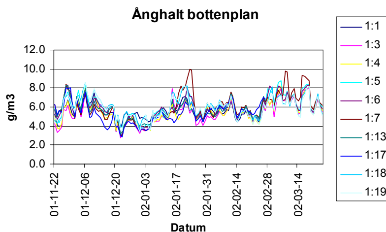
Figur 7.9 Dygnsmedelånghalt bottenplan
