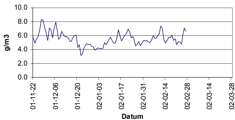
Ånghalt Rum 1:13
