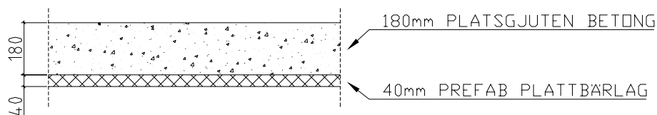
Figur 3.5 Bjälklag 220 mm.
