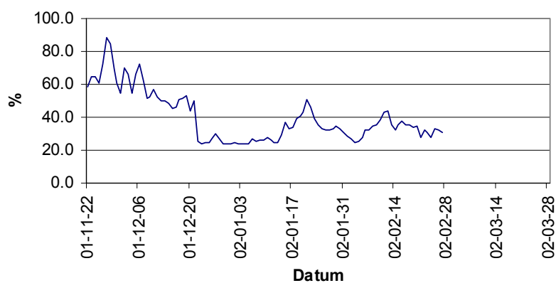
RF Rum 1:13
