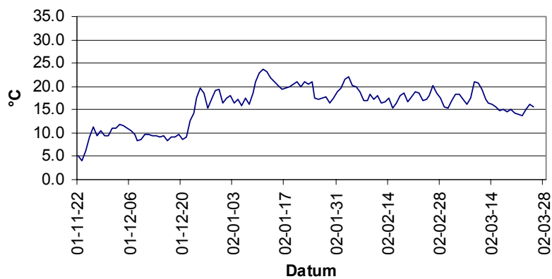
Temperatur Rum 1:19
