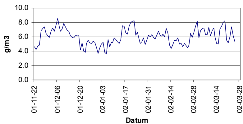
Ånghalt Rum 1:18
