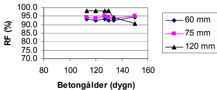
Betong-RF Rum 1:17
