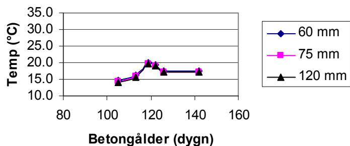
Betongtemperatur Rum 1:12
