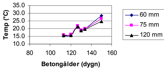
Betongtemperatur Rum 1:17
