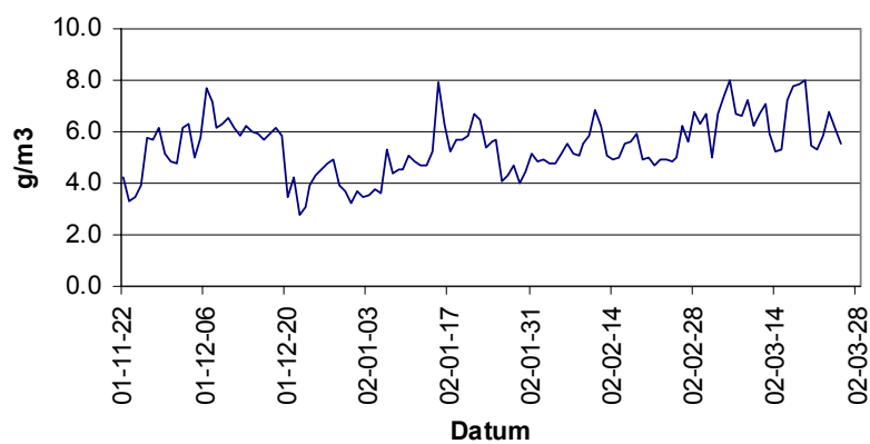
Ånghalt Rum 1:3
