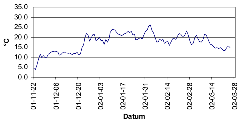
Temperatur Rum 1:18
