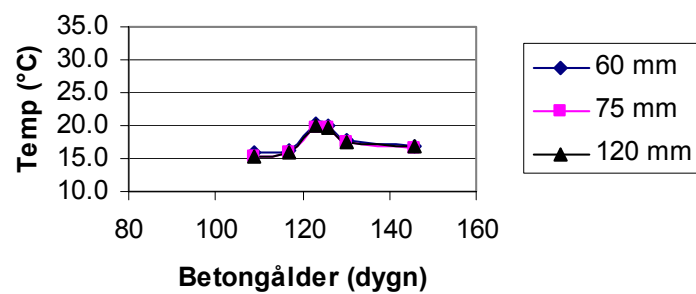
Betongtemperatur Rum 1:11
