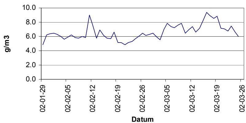
Ånghalt Rum 2:19
