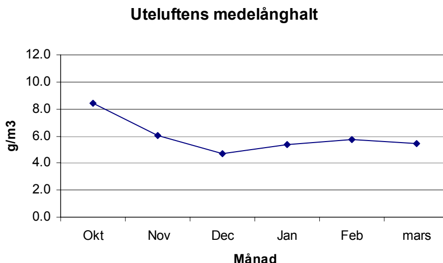
Figur 7.4 Månadsmedelånghalten utomhus
