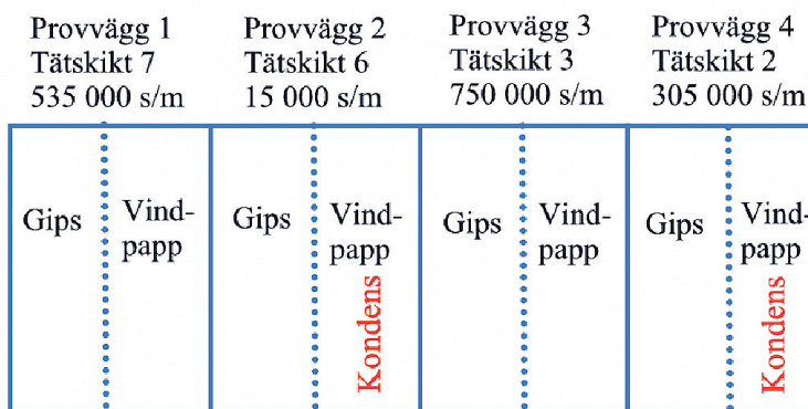
Figur 6: Resultat av väggar utan plastfolie med kallt klimat på utsidan och duschning två gånger per dag under cirka tre månaders tid.
